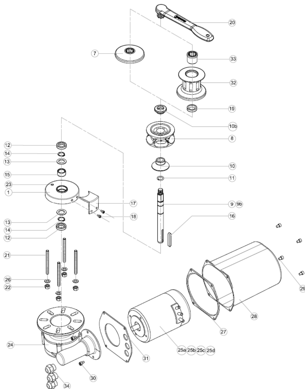
Esploso Smart R-1 1000W
